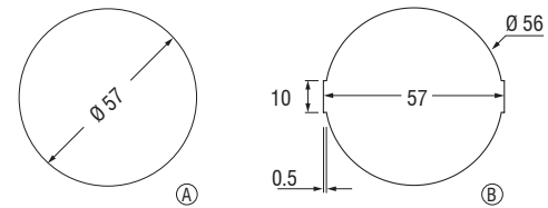
Foro di incasso / Recessed hole / Einbaumaße
